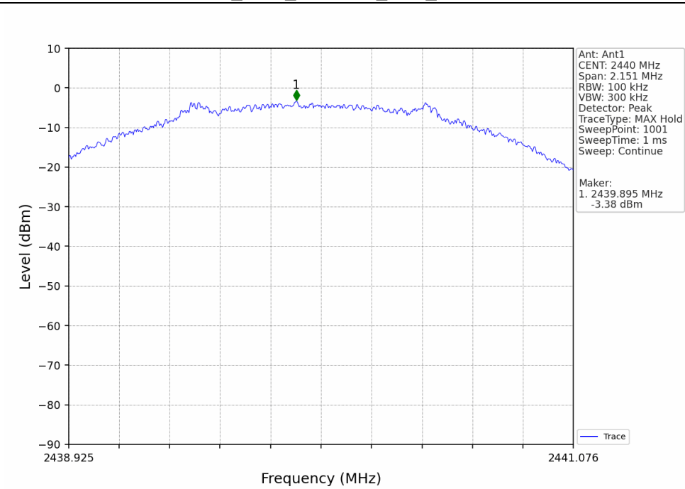
2M_MCH_2440MHz_Ant1_NTNV
