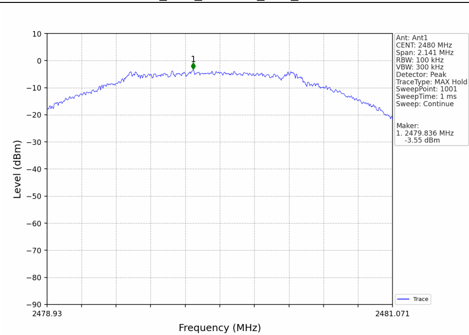
2M_HCH_2480MHz_Ant1_NTNV
