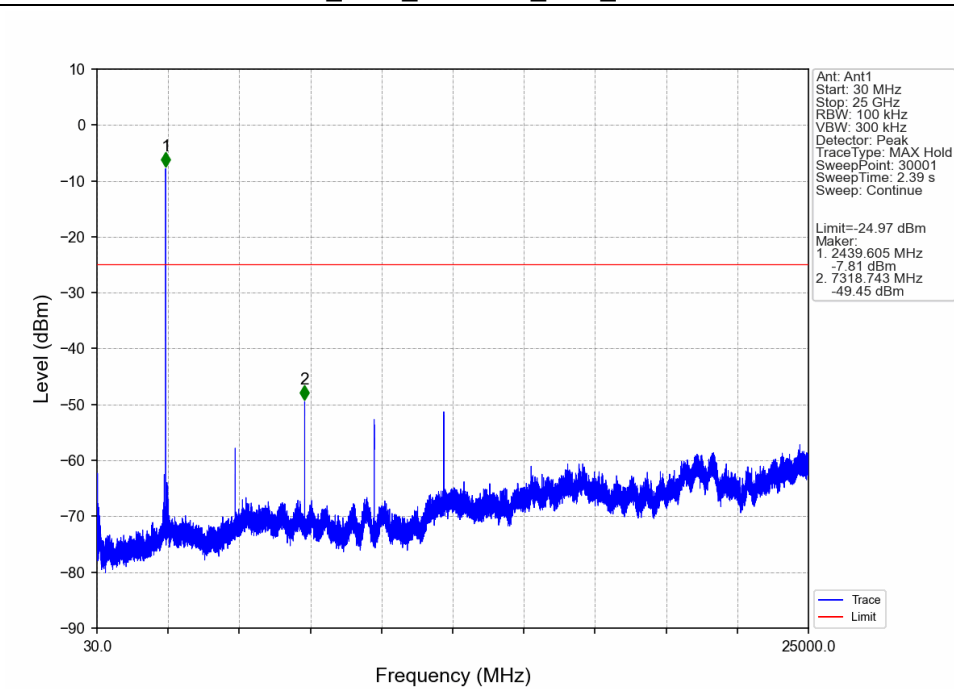
2M_MCH_2440MHz_Ant1_NTNV
