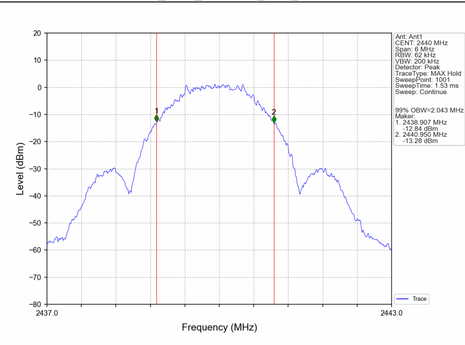
2M_MCH_2440MHz_Ant1_NTNV
