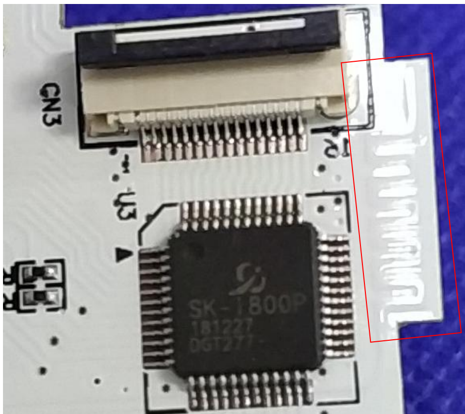
ANTENNA
