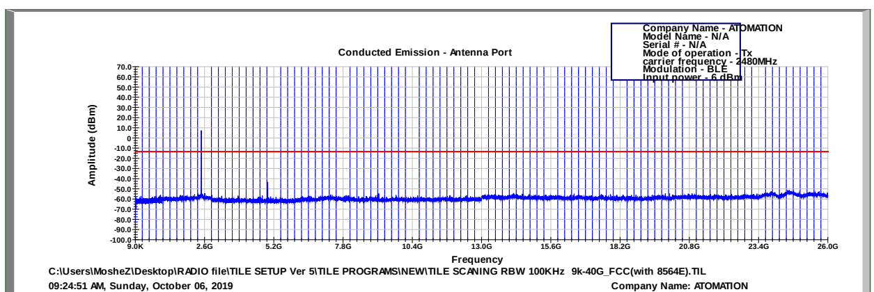
Figure 36 2480.0 MHz, BLE
