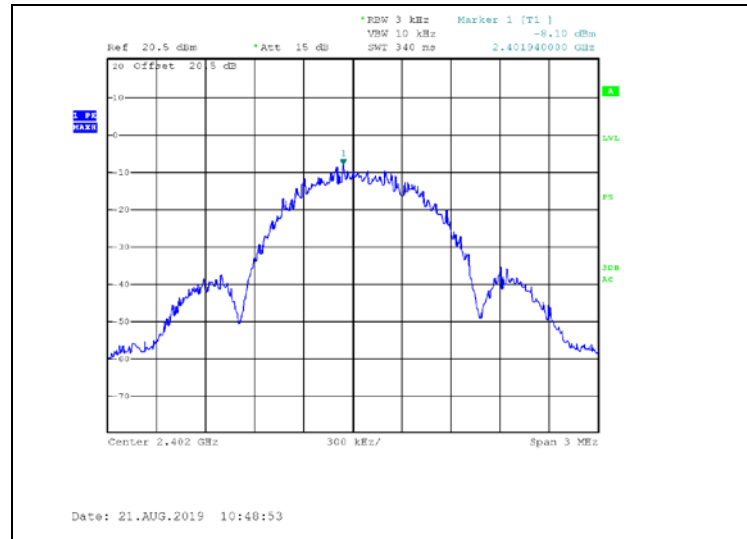
Figure 25. 2402.0 MHz, BLE
