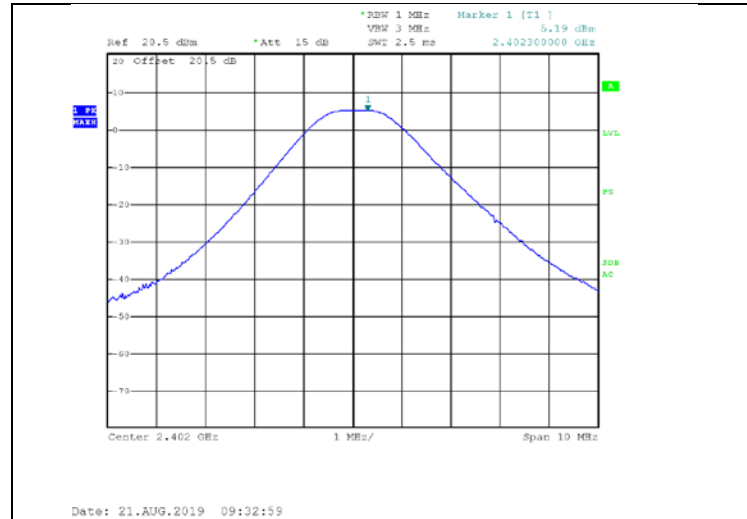
Figure 16. 2402.0 MHz, BLE
