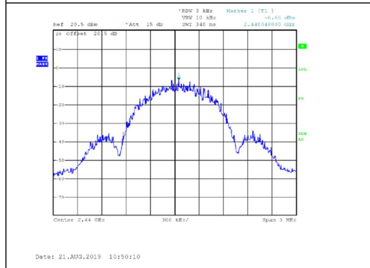
Figure 26. 2440.0 MHz, BLE
