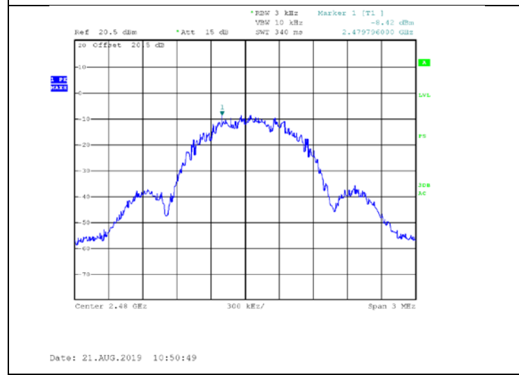
Figure 27. 2480.0 MHz, BLE
