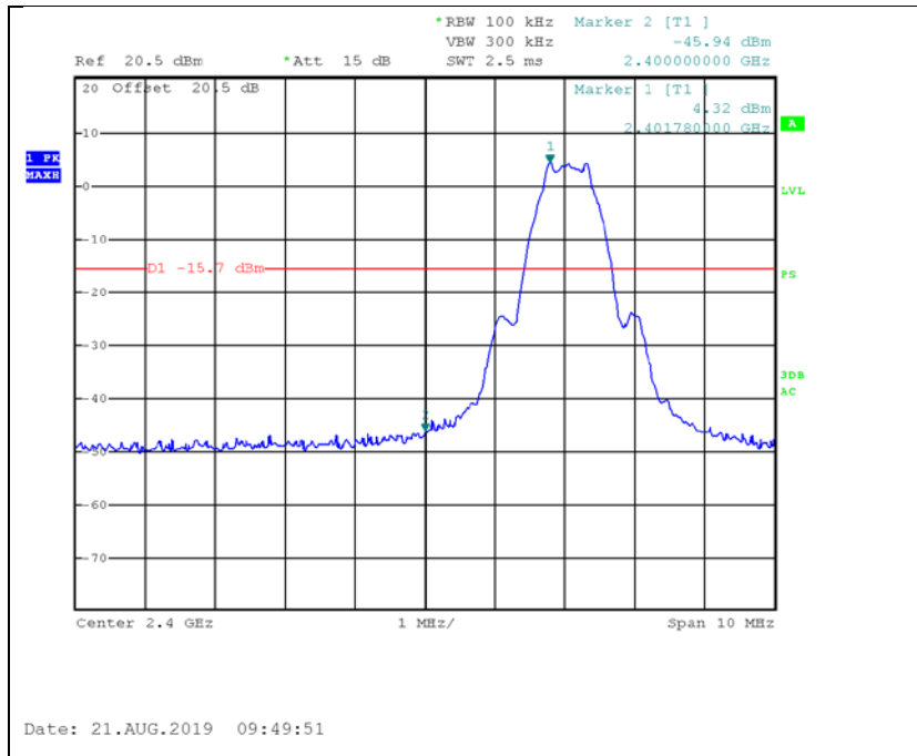
Figure 21. 2402.0 MHz, BLE
