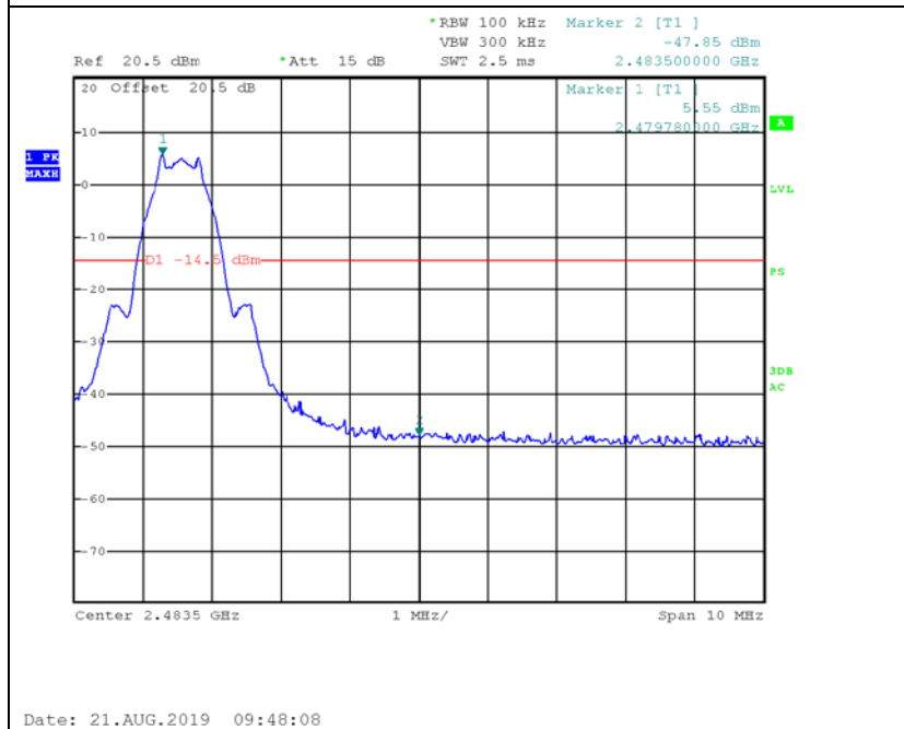
Figure 22. 2480.0 MHz, BLE
