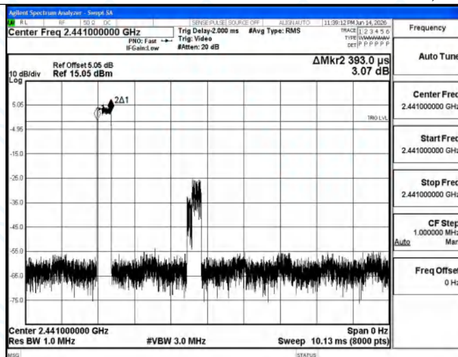
2DH3_Ant1_Hop
