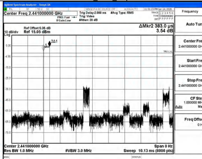
DH3_Ant1_Hop
