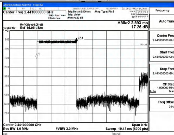
3DH1_Ant1_Hop
