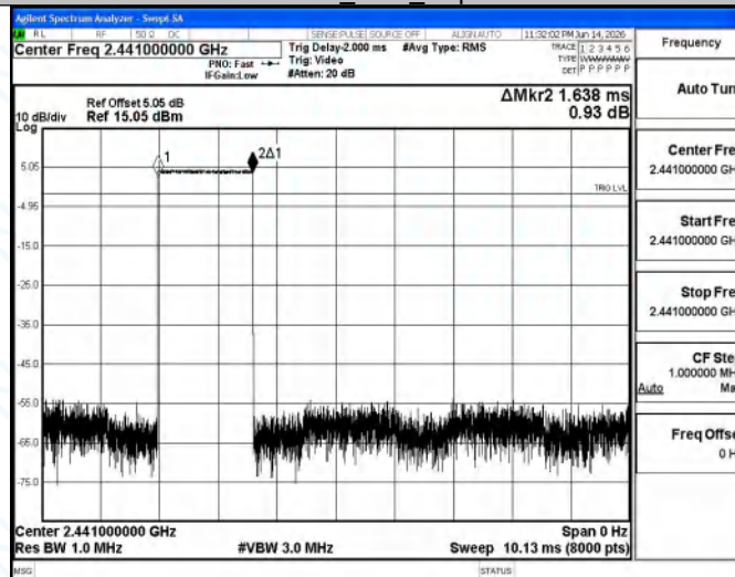
DH5_Ant1_Hop
