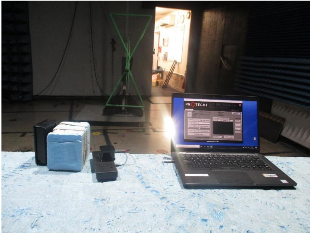
EUT Upright
