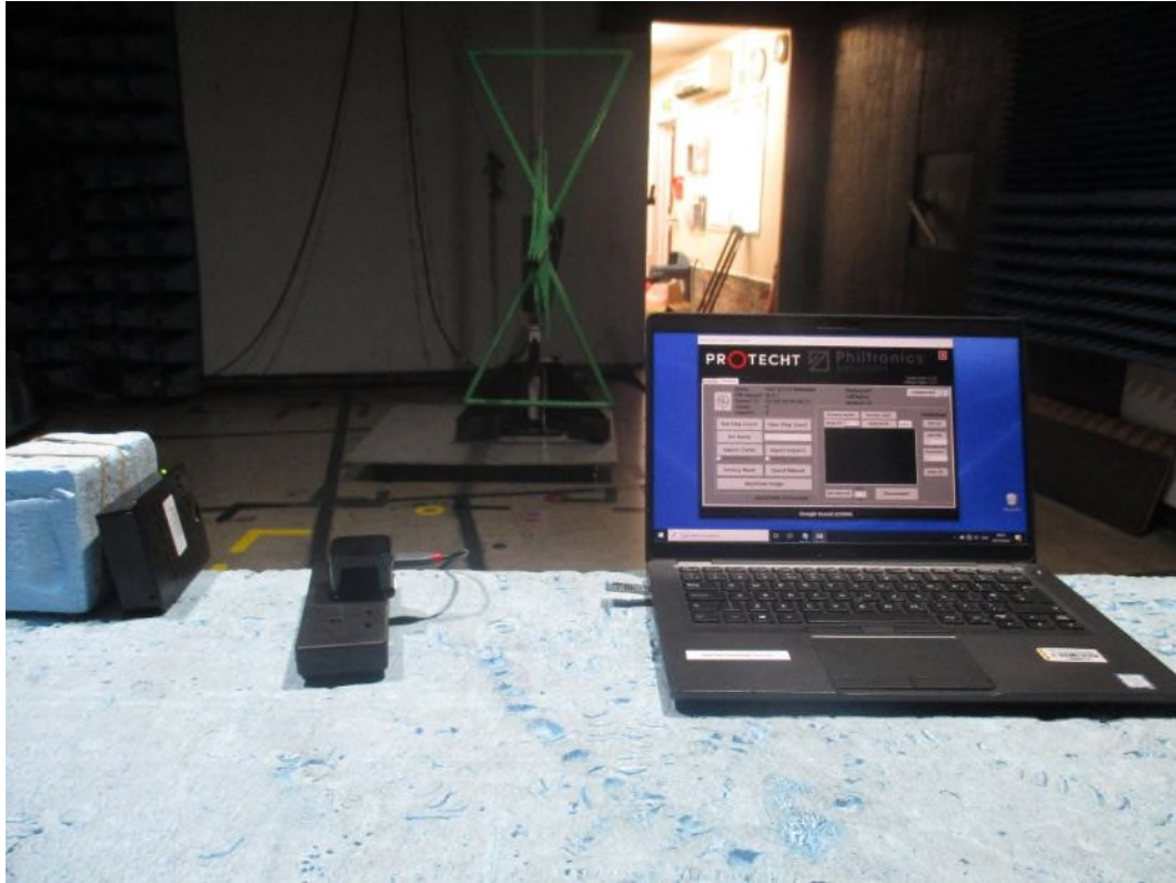
EUT Side
