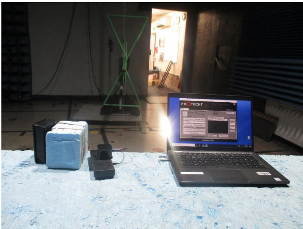
EUT Upright
