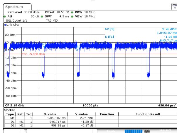
802.11ac40_5190MHz
