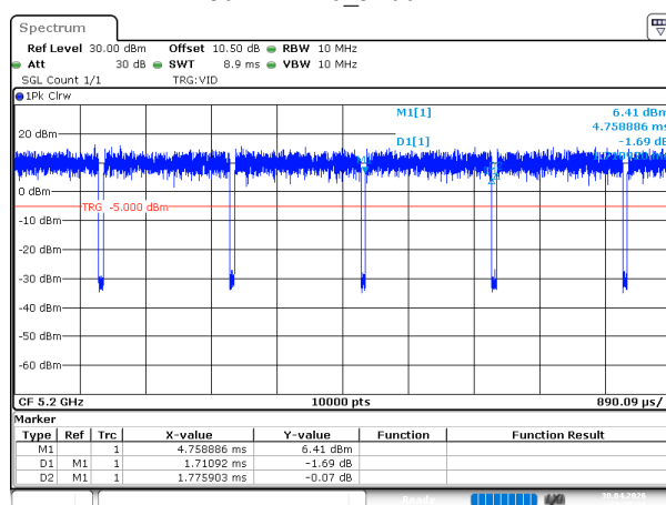
802.11ac20_5200MHz
