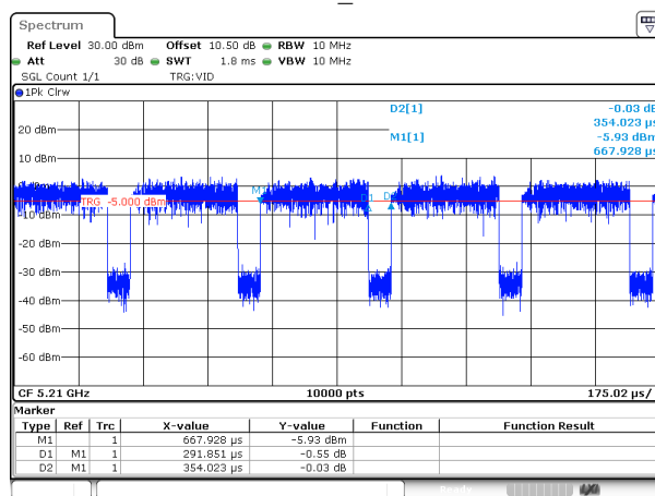
802.11ac80_5210MHz
