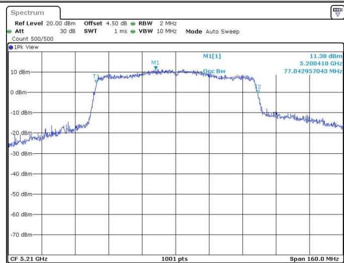
11AC80SISO_Ant1_5210
