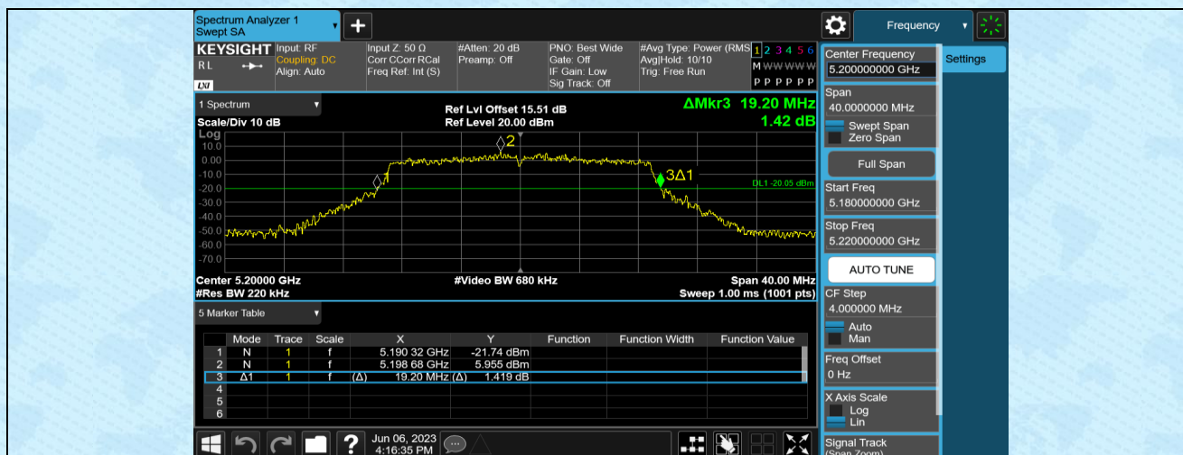
11N20MIMO-Ant2-5200
