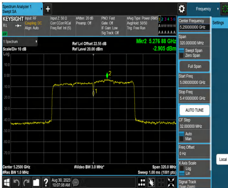
11AX160MIMO_Ant2_5250_UNII-2A
