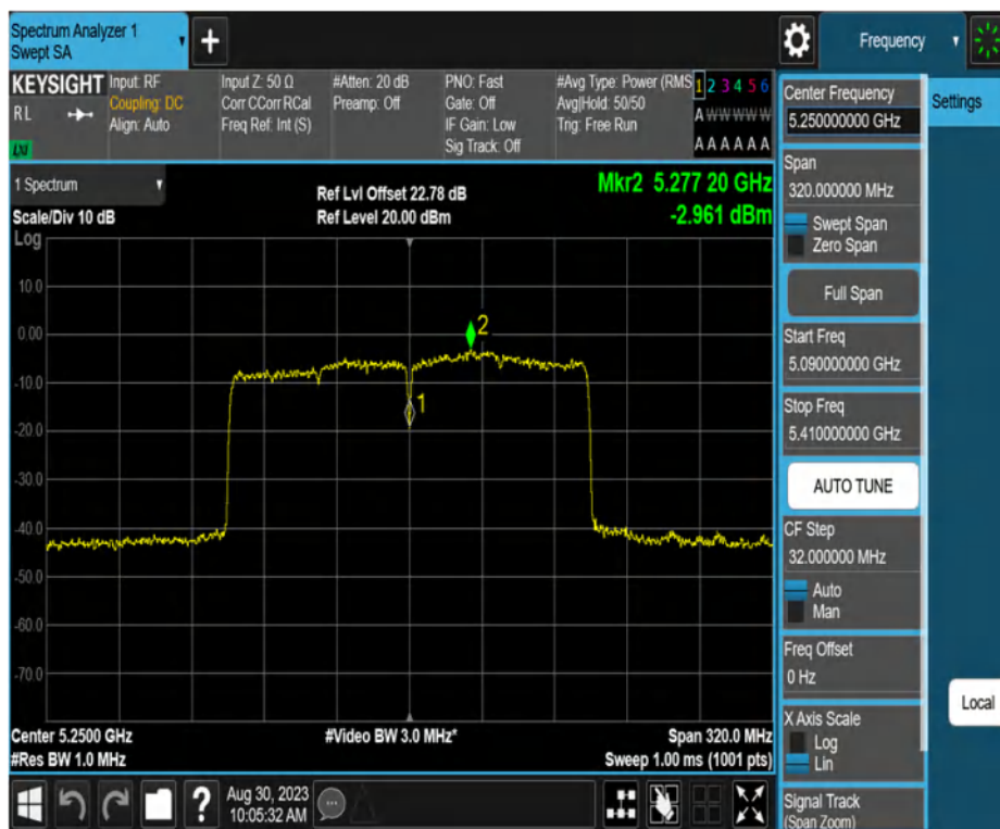
11AX160MIMO_Ant2_5250_UNII-2A
