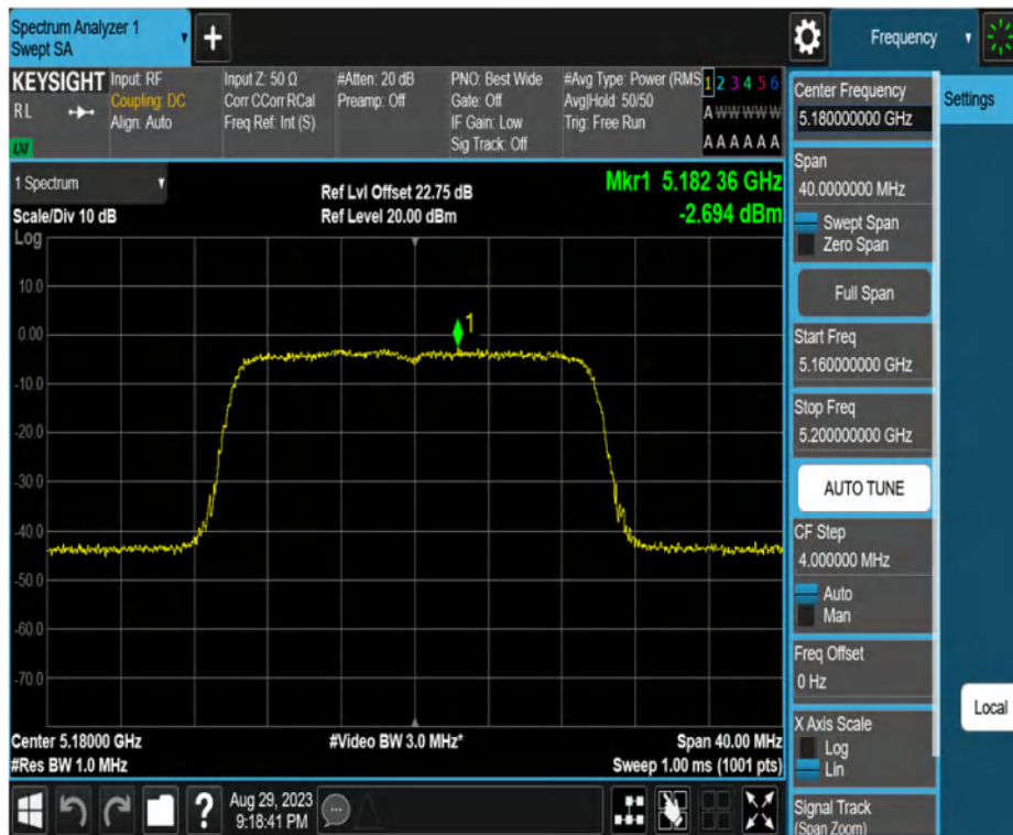
11AX20MIMO_Ant2_5180
