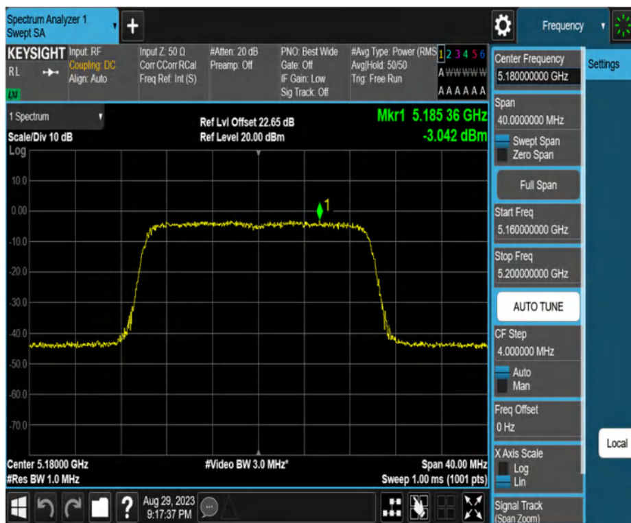
11AX20MIMO_Ant2_5180
