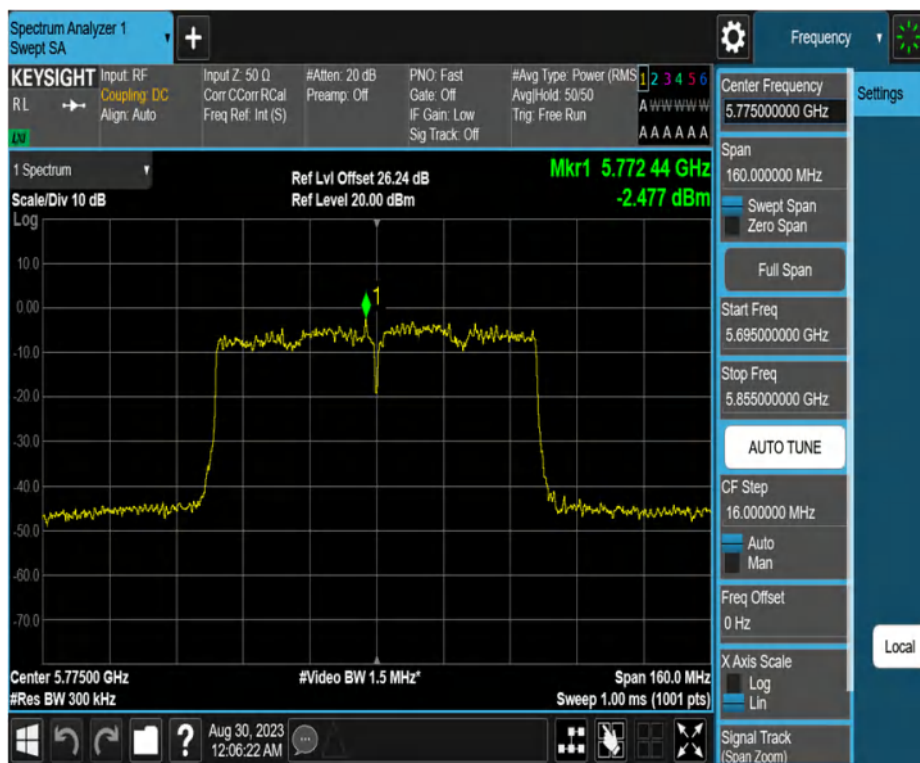
11AC80MIMO_Ant2_5775
