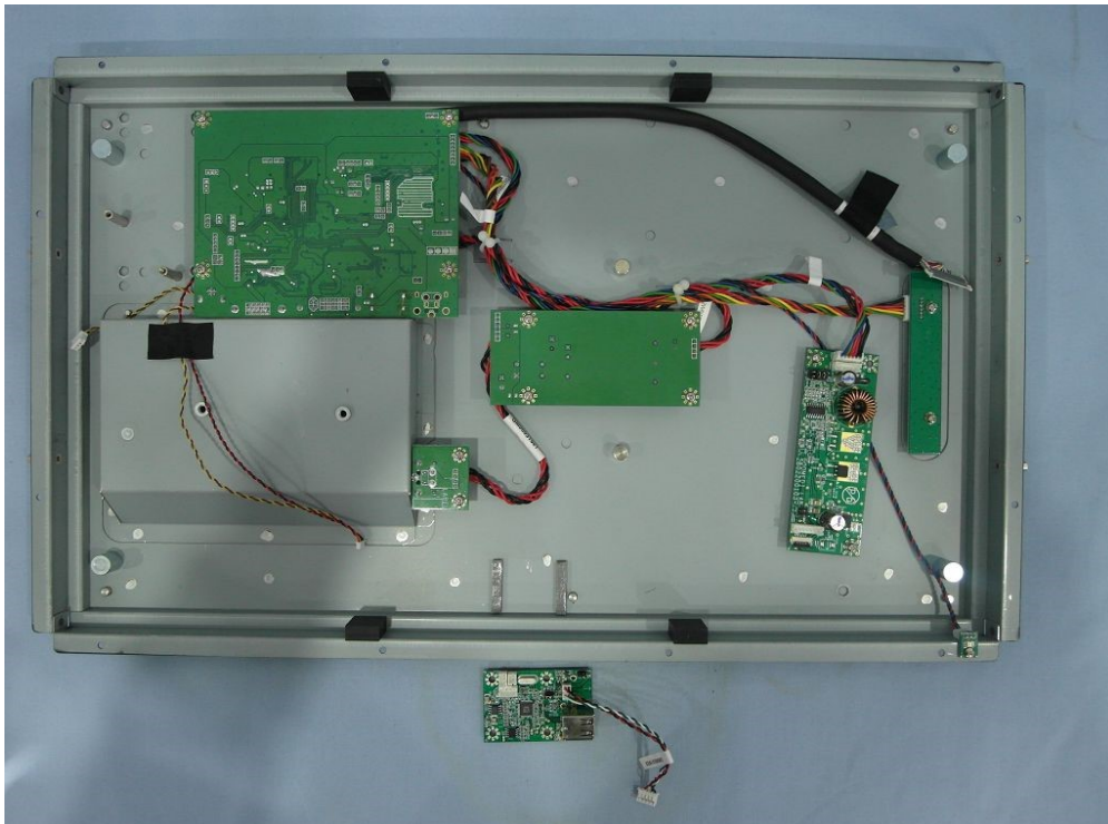
(19) EUT Photo
