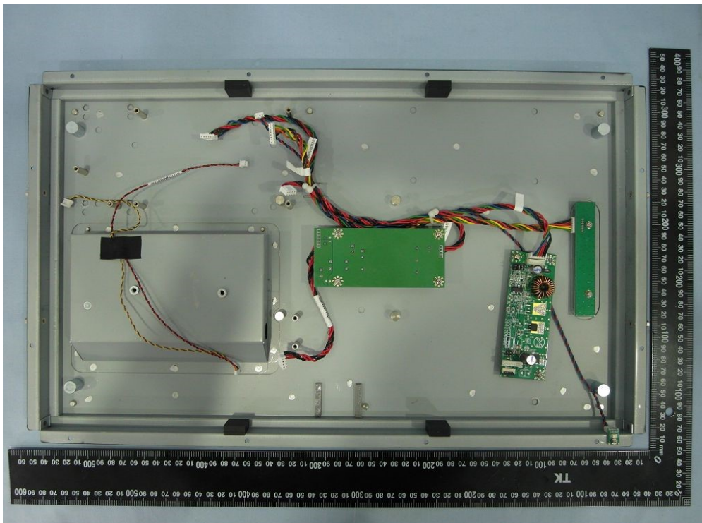
(33) EUT Photo
