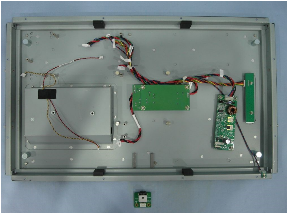
(31) EUT Photo
