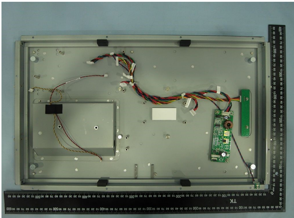
(37) EUT Photo
