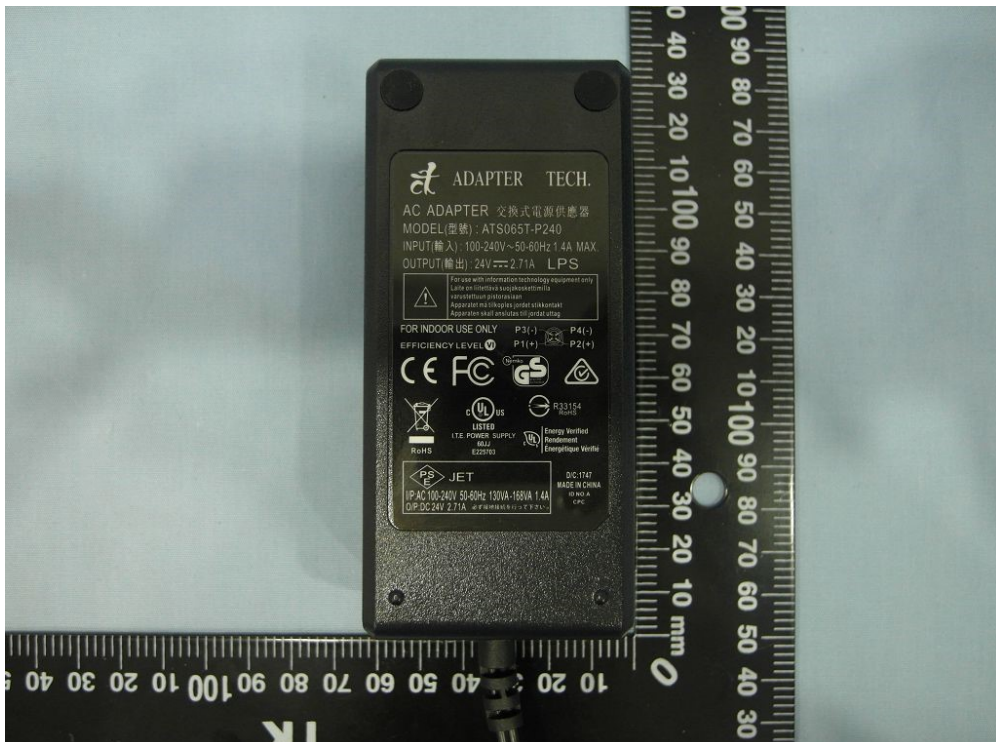
(53) EUT Photo
