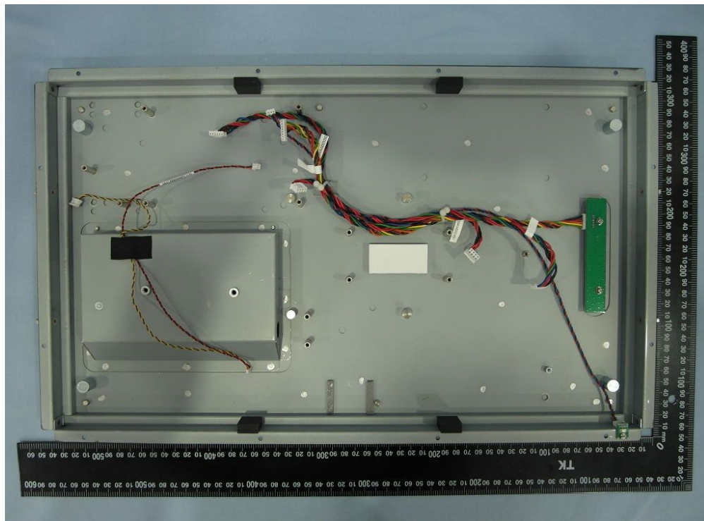
(41) EUT Photo
