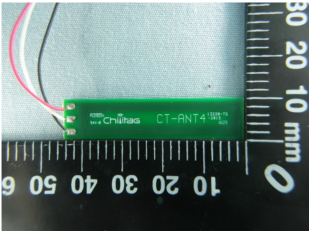
(47) EUT Photo
