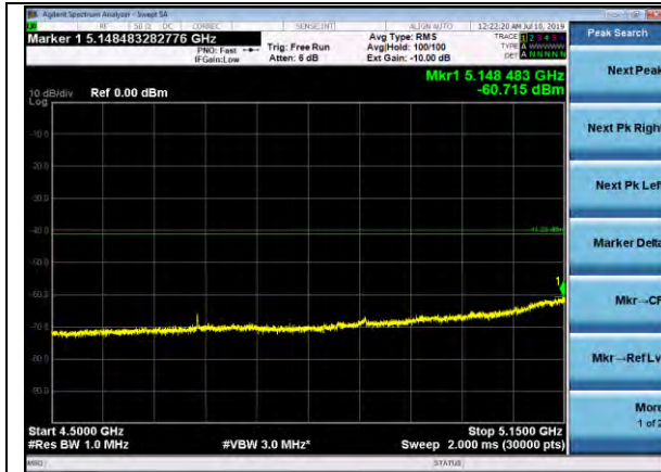
MCS0 LBE
