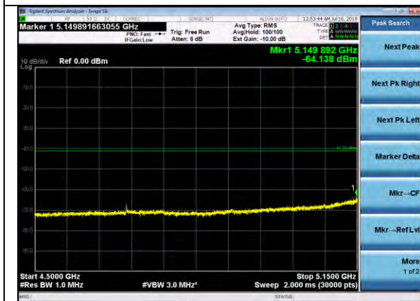
MCS7 LBE
