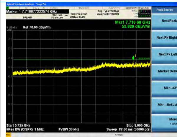
5.725 – 8 GHz
