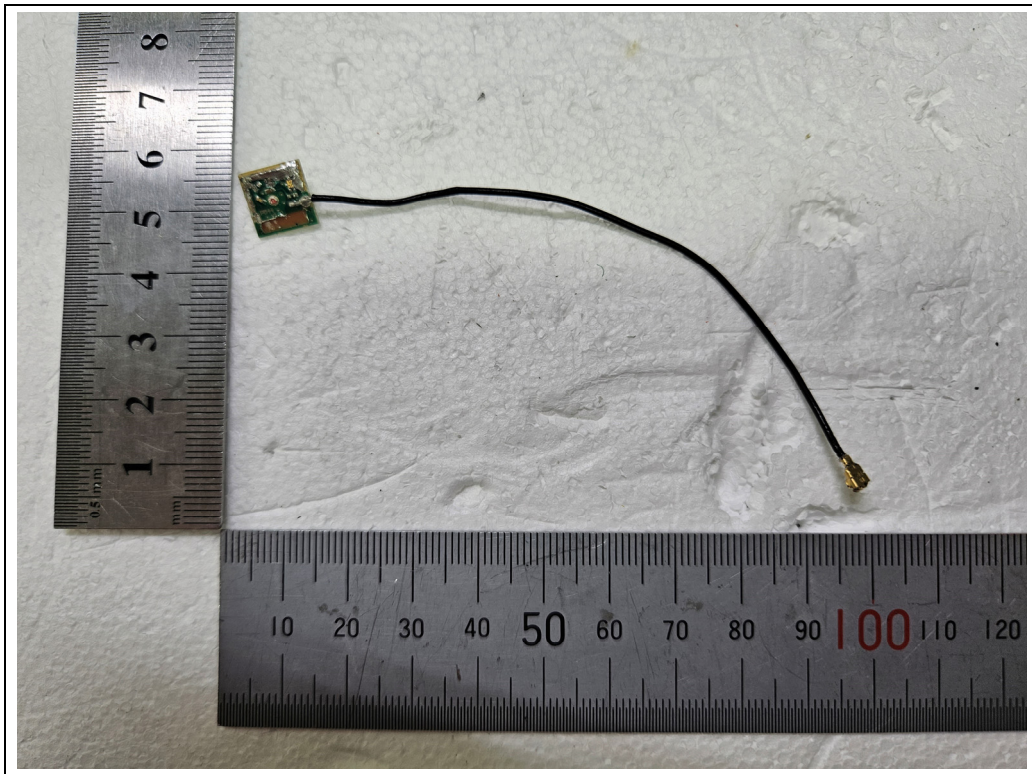
<GNSS Antenna>
