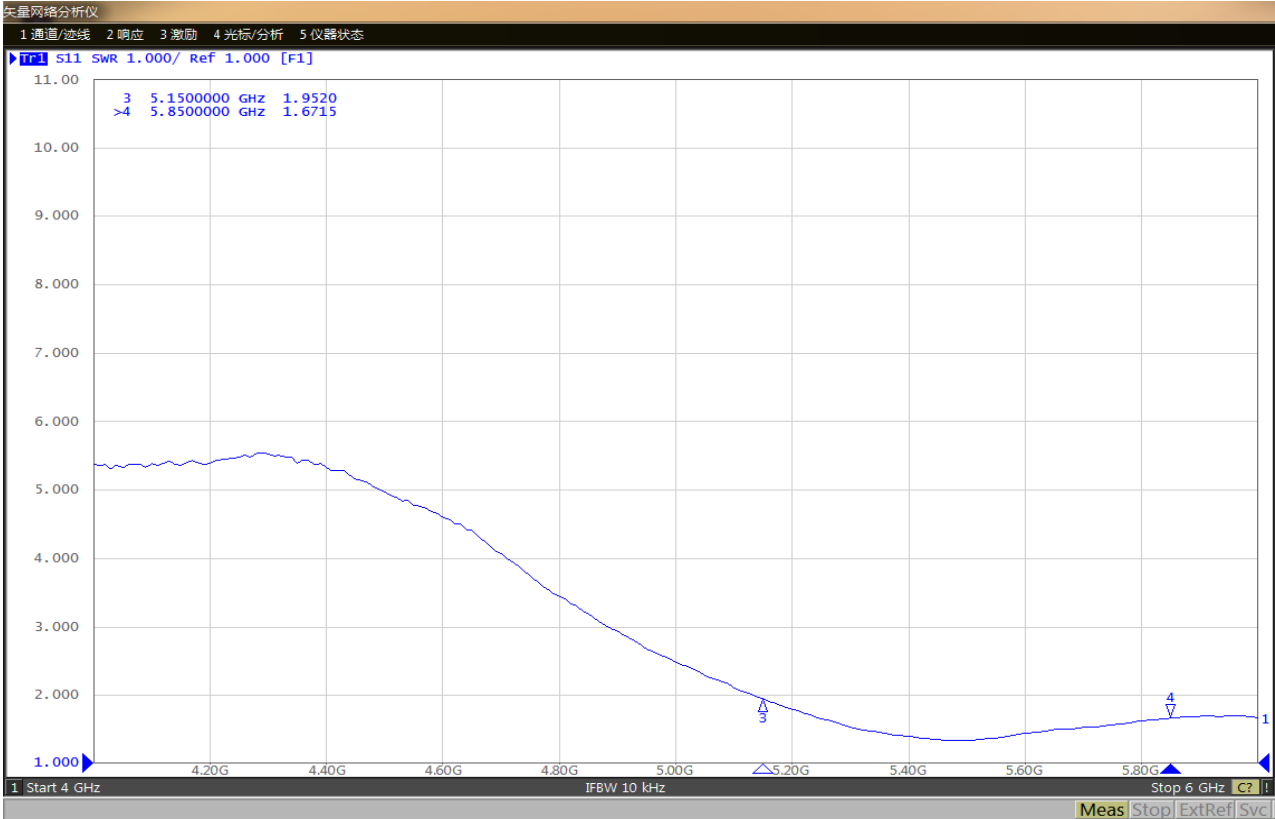
驻波比测试
