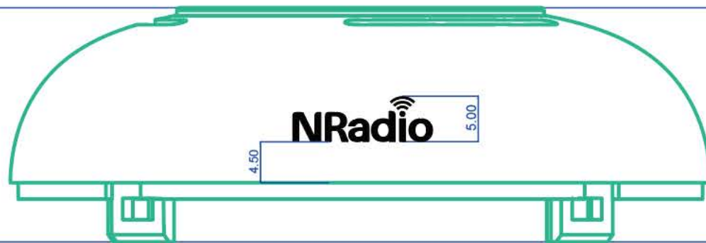
正视图
