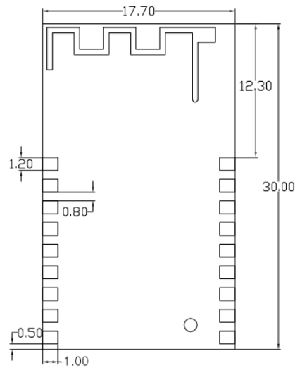
Fig 3 - Module Dimensions
