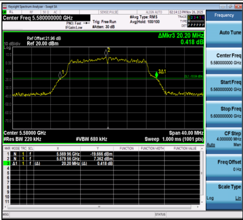
11A-Ant1-5580
