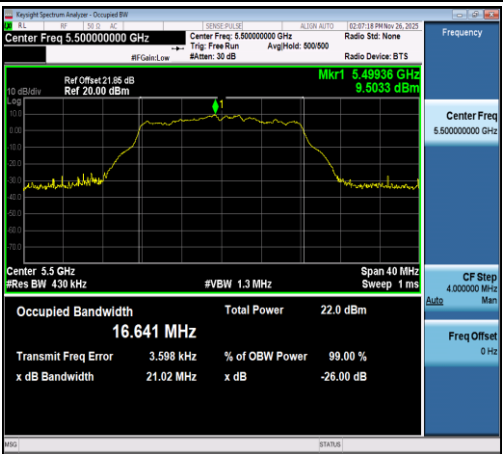
11A-Ant1-5500
