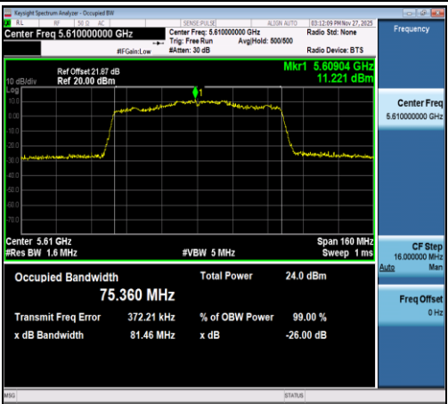
11AC80SISO-Ant1-5610
