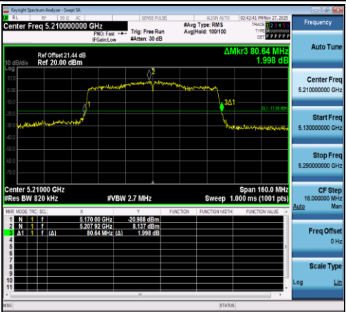
11AC80SISO-Ant1-5210
