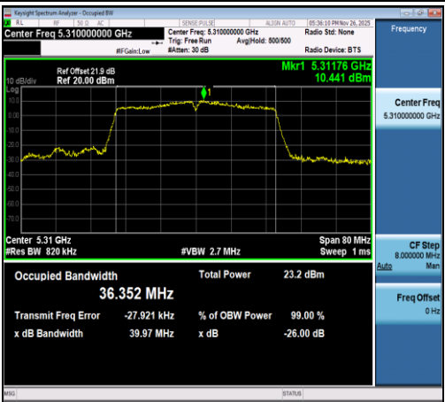
11N40SISO-Ant1-5310
