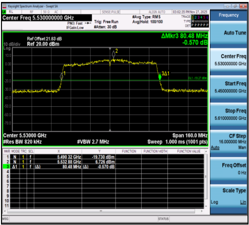
11AC80SISO-Ant1-5530
