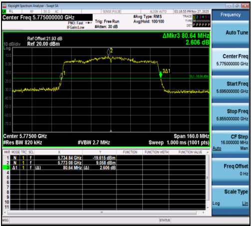
11AC80SISO-Ant1-5775
