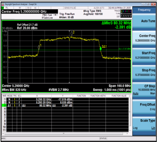
11AC80SISO-Ant1-5290
