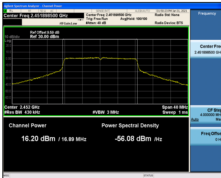
11G_Ant1_2457
