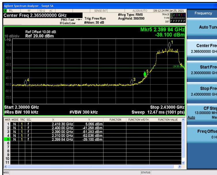
11G_Ant1_Low_2422
