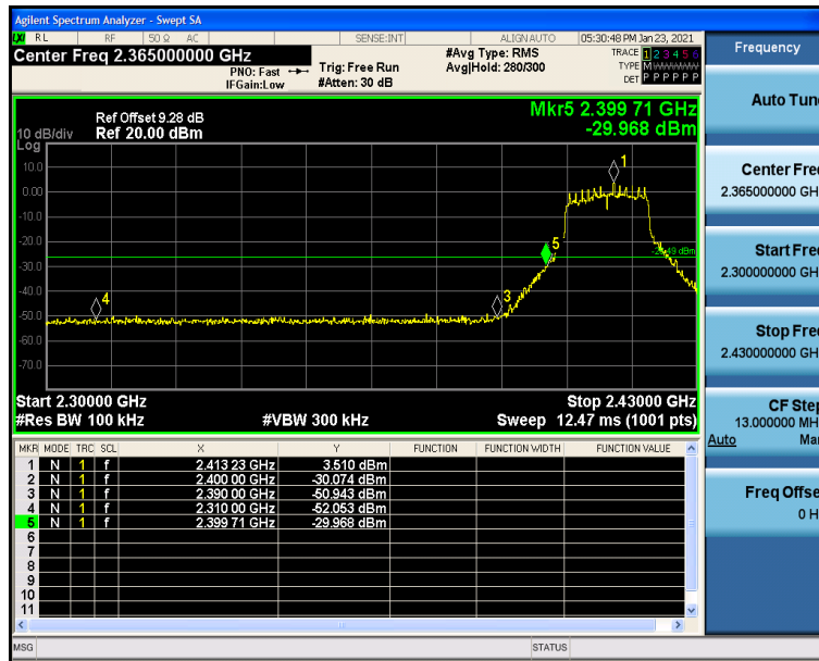
11G_Ant1_Low_2417
