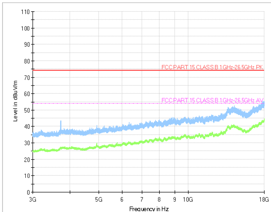
Worst case-11b-iso-CH_2462
