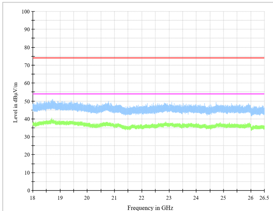
Worst case-11b-iso-CH_2462
