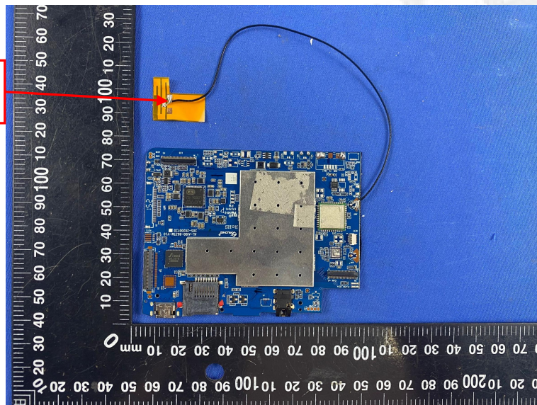
Bluetooth/WiFi Antenna
