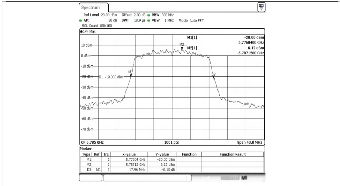
11A-Ant0-5785
