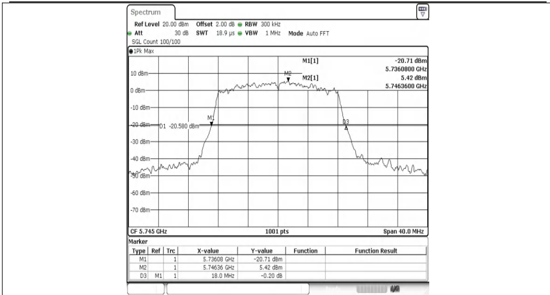
11A-Ant0-5745
