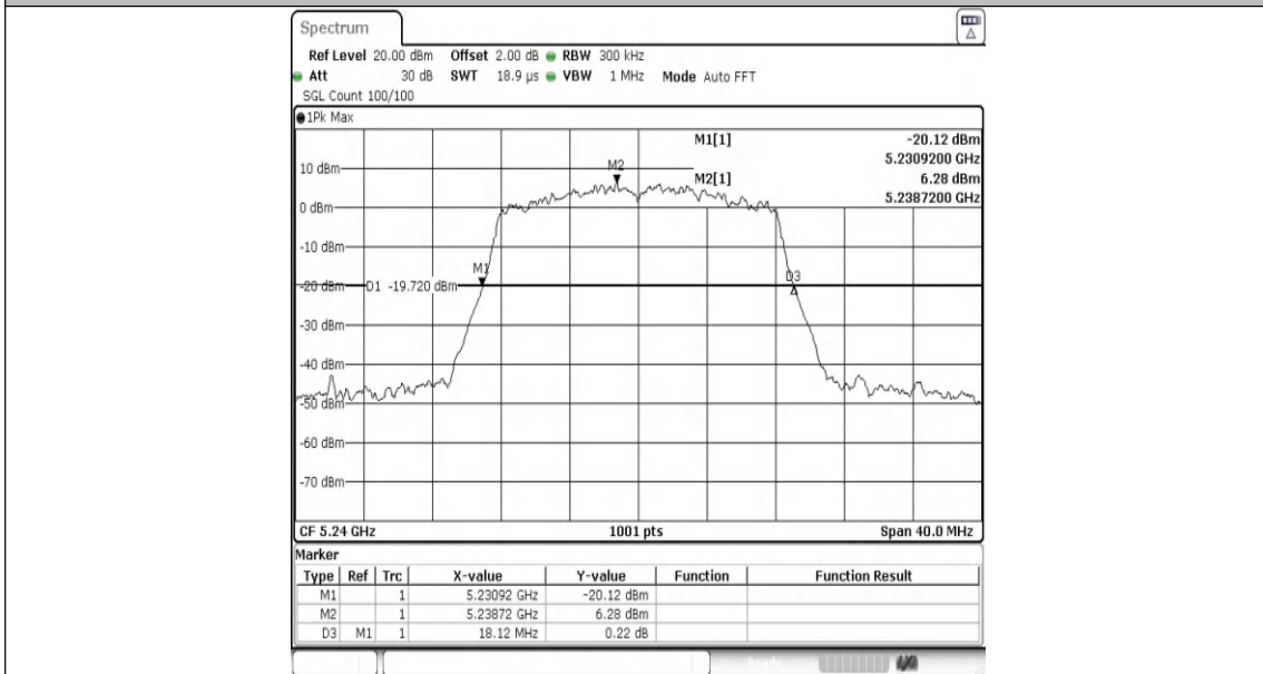
11A-Ant0-5240
