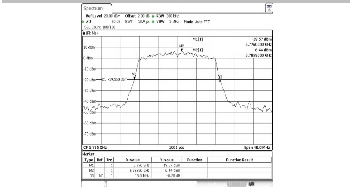
11A-Ant0-5785
