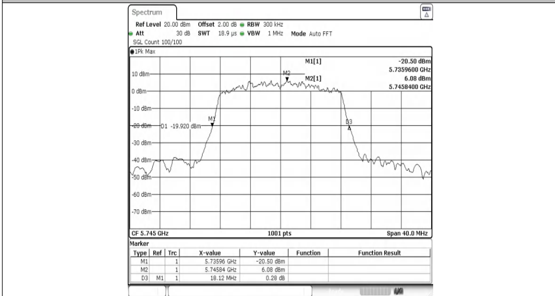
11A-Ant0-5745
