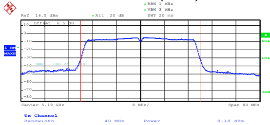
802.11n(HT40)
