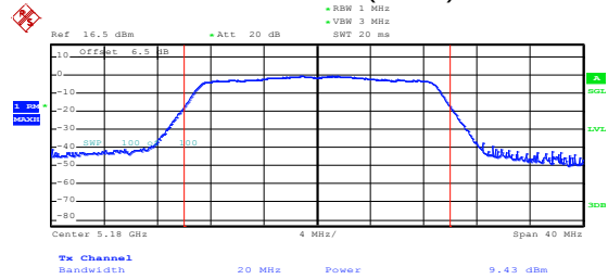
802.11ac(HT20)
