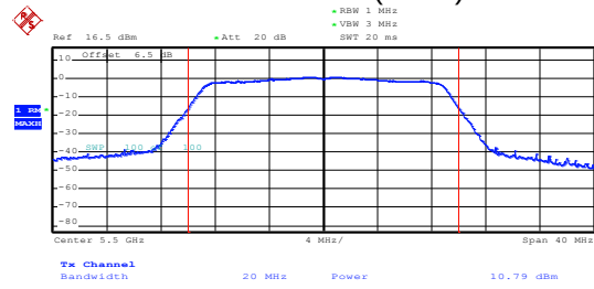
802.11ac(HT20)
