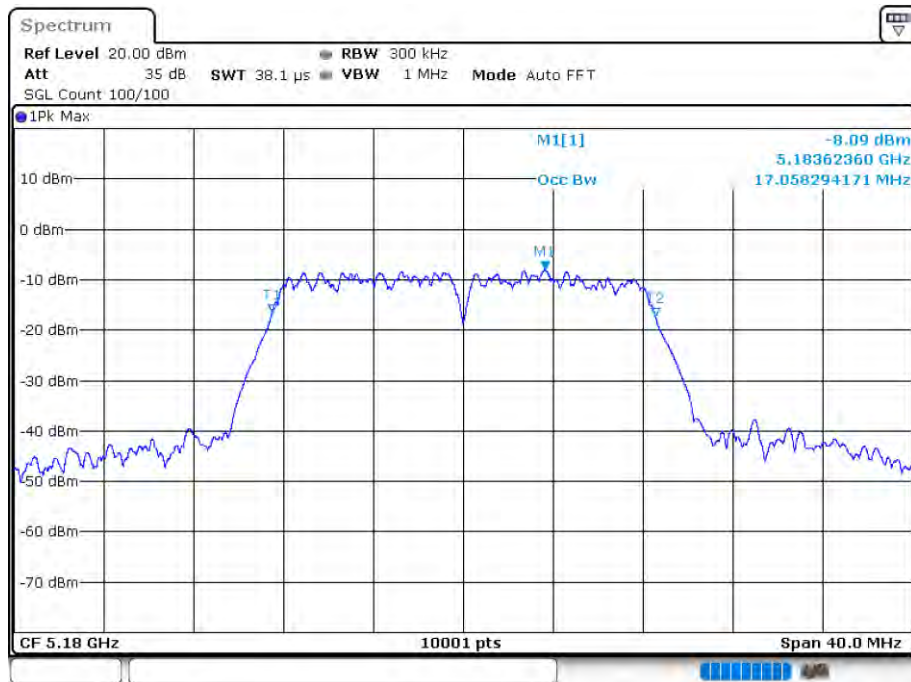
OBW NVNT 802.11a 5180MHz Ant1
