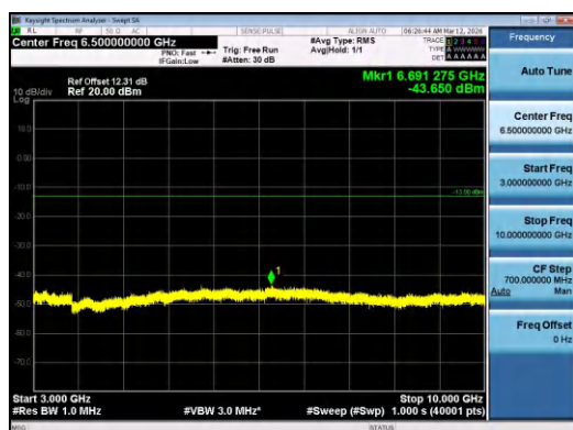
Band12-3MHz-QPSK-23095-15RB#0-3000~10000-PA
