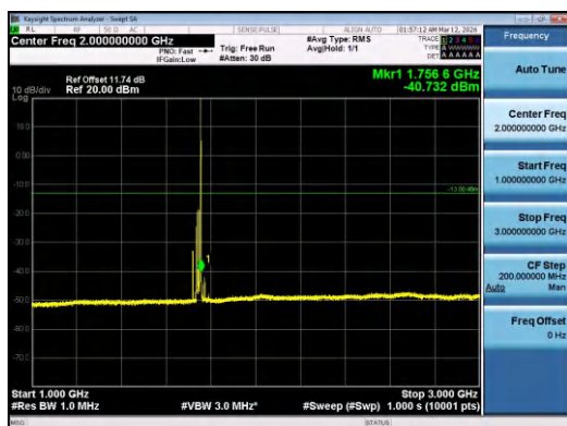
Band4-20MHz-QPSK-20300-1RB#99-1000~3000-PAS
