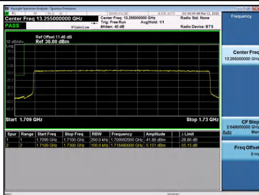
Band4-20MHz-QPSK-20050-100RB#0-PASS
