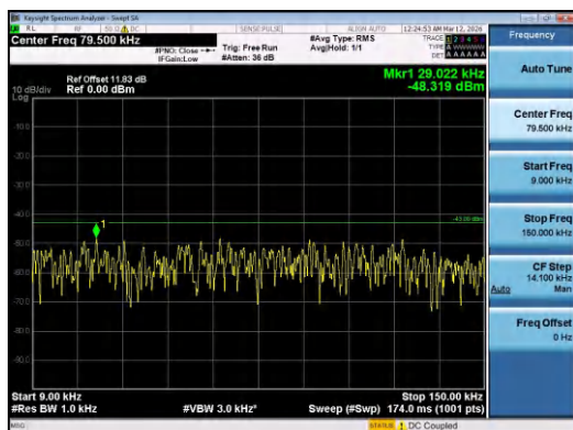
Band4-10MHz-QPSK-20175-50RB#0-0.009~0.15-PAS
