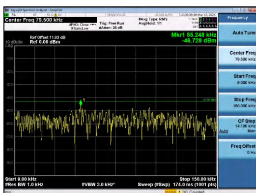
Band4-10MHz-QPSK-20350-50RB#0-0.009~0.15-PAS
