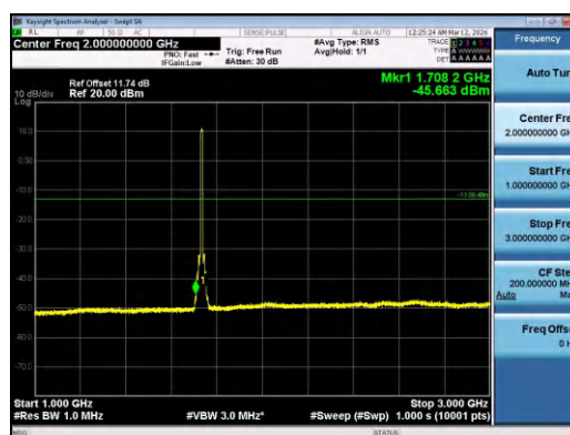
Band4-10MHz-QPSK-20175-50RB#0-1000~3000-PAS
