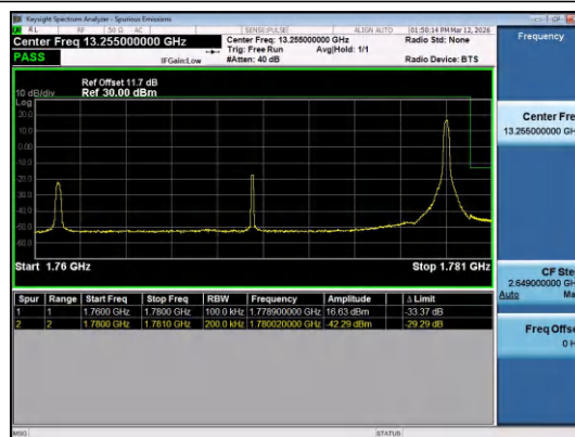
Band66-20MHz-QPSK-132572-1RB#99-PASS
