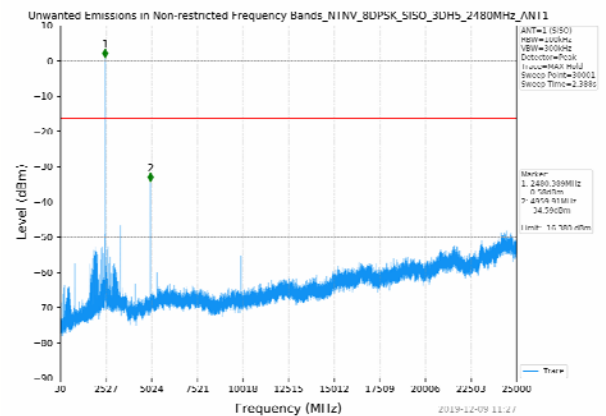
30MHz-25GHz CH78
