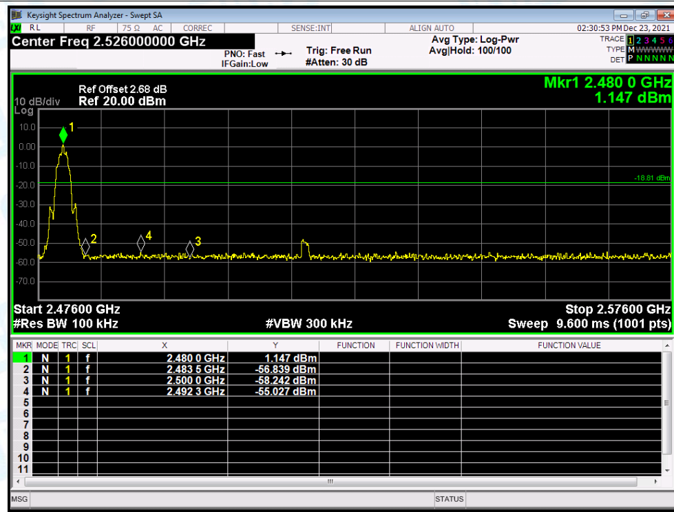
Band Edge NVNT BLE 2Mbps 2480MHz Ant1 Emission
