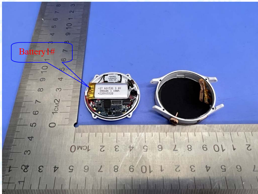
Photo 5 Battery parameters
