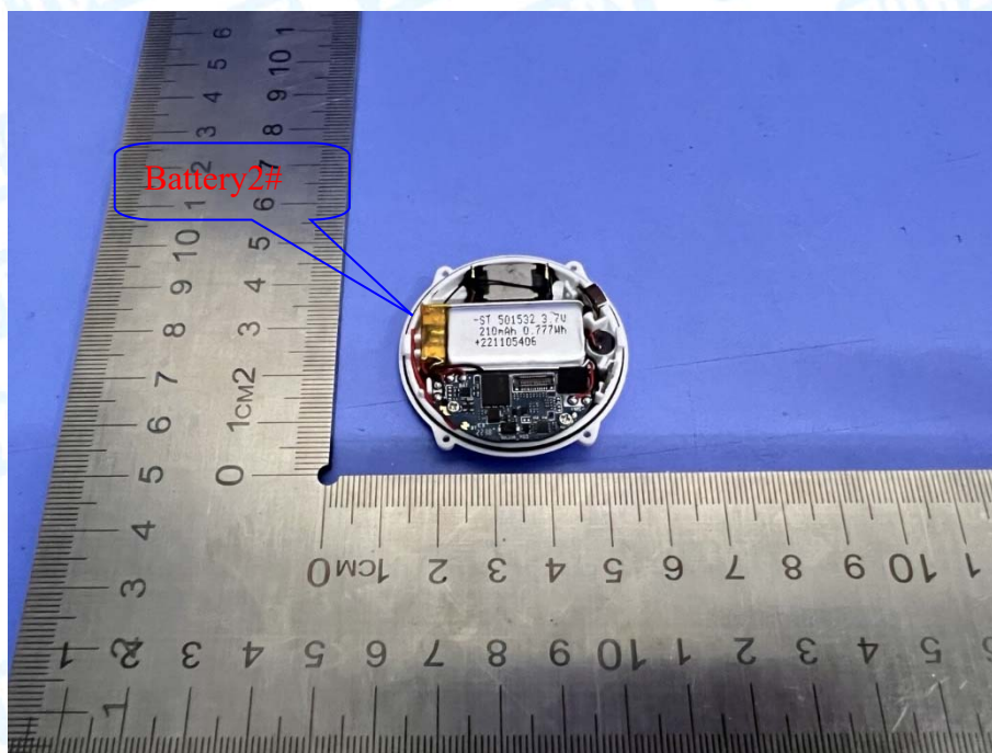
Photo 5 Battery parameters
