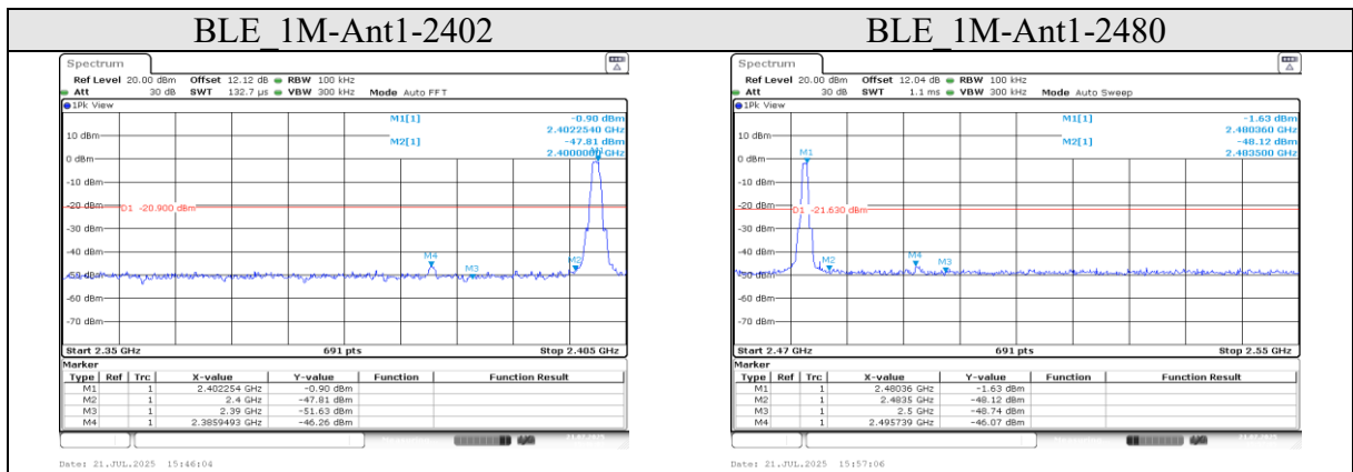
Figure 2: Band Edge
