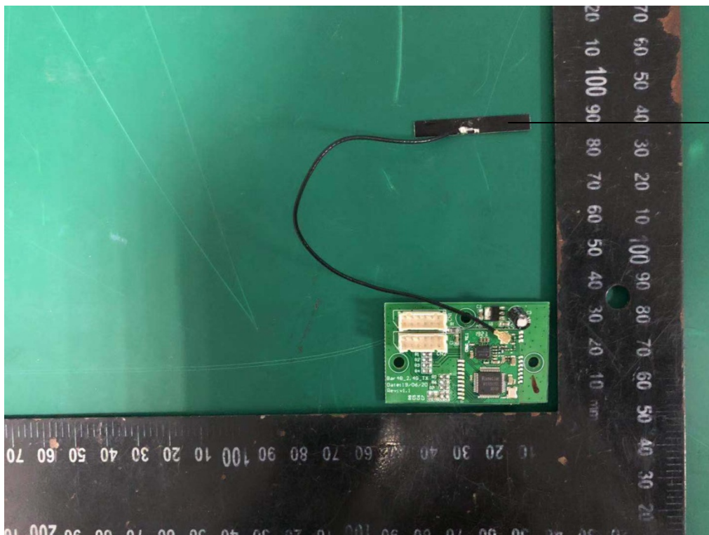
2.4G Antenna
