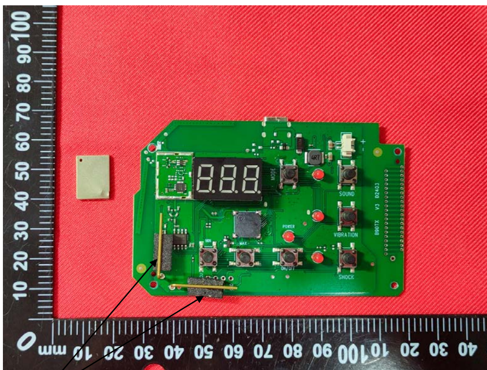
2.4G Antenna
