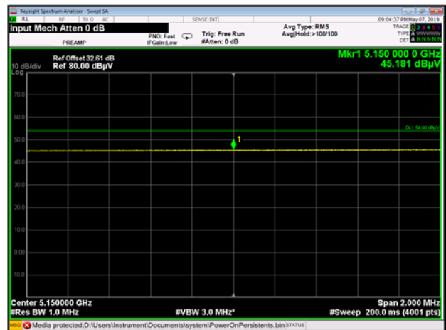
Band I 11ac20 CH36 AV
