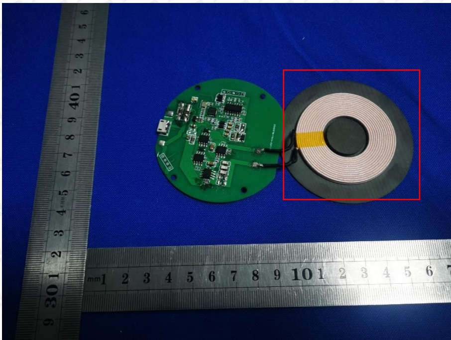
4 EUT ANTENNA:
