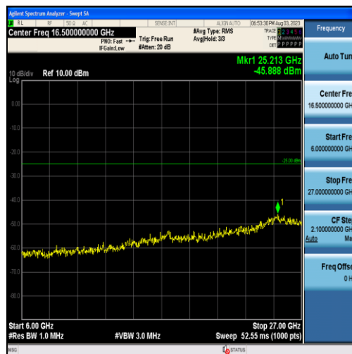
Band7-10MHz-16QAM-20800-50RB#0-Range3:6000~27000MHz
