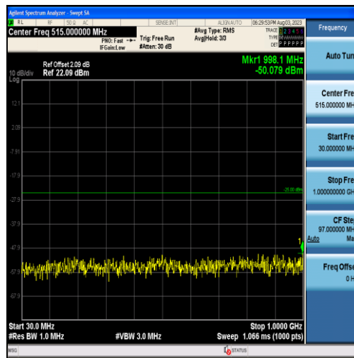
Band7-10MHz-QPSK-20800-50RB#0-Range1:30~1000MHz
