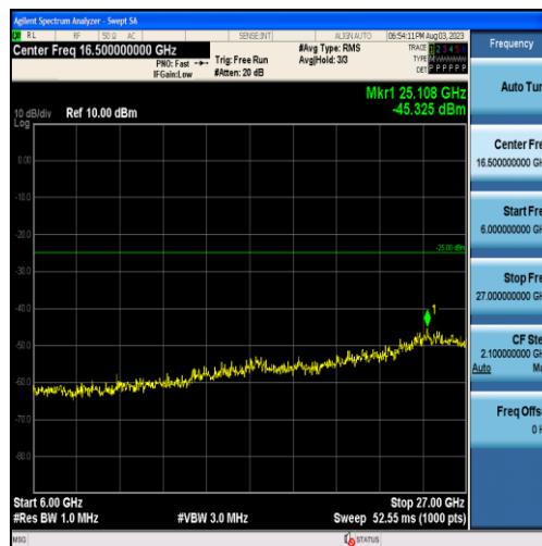
Band7-10MHz-16QAM-21100-50RB#0-Range3:6000~27000MHz
