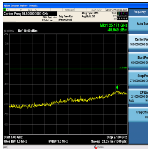
Band7-10MHz-QPSK-21100-50RB#0-Range3:6000~27000MHz
