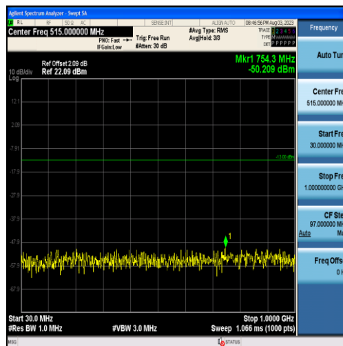
Band25-1.4MHz-QPSK-26365-6RB#0-Range1:30~1000MHz
