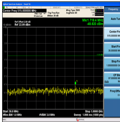
Band25-1.4MHz-QPSK-26047-6RB#0-Range1:30~1000MHz
