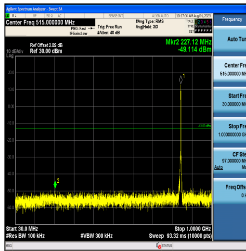
Band26-3MHz-QPSK-27025-15RB#0-Range1:30~1000MHz
