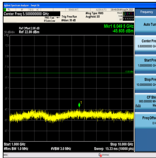
Band26-3MHz-QPSK-26775-15RB#0-Range2:1000~10000MHz
