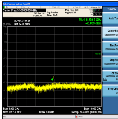
Band26-5MHz-QPSK-26765-25RB#0-Range2:1000~10000MHz
