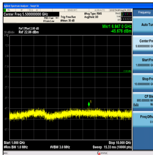
Band26-10MHz-QPSK-26740-50RB#0-Range2:1000~10000MHz
