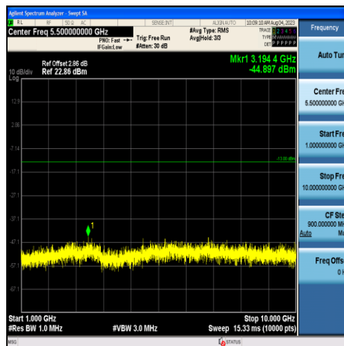
Band26-1.4MHz-QPSK-26797-6RB#0-Range2:1000~10000MHz
