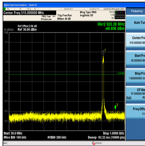
Band26-10MHz-QPSK-26740-50RB#0-Range1:30~1000MHz
