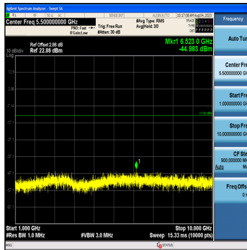
Band26-3MHz-QPSK-27025-15RB#0-Range2:1000~10000MHz
