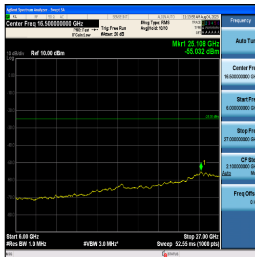
Band38-5MHz-QPSK-38225-25RB#0-Range3:6000~27000MHz
