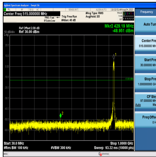
Band26-10MHz-QPSK-26990-50RB#0-Range1:30~1000MHz
