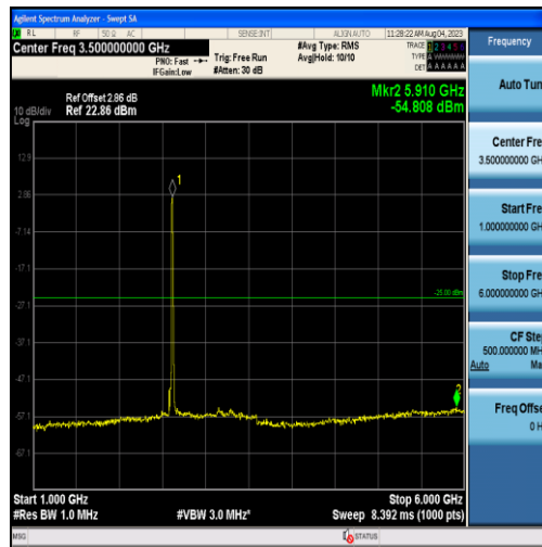
Band38-10MHz-QPSK-38200-50RB#0-Range2:1000~6000MHz
