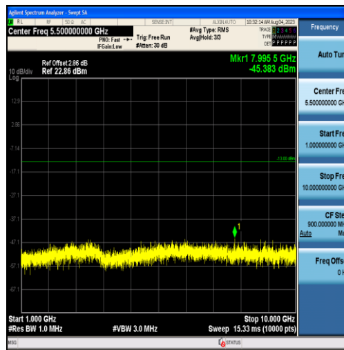
Band26-10MHz-QPSK-26840-50RB#0-Range2:1000~10000MHz
