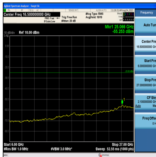
Band38-10MHz-QPSK-38000-50RB#0-Range3:6000~27000MHz
