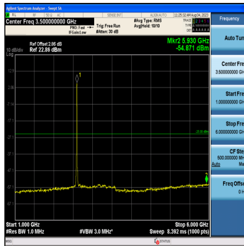
Band38-10MHz-QPSK-38000-50RB#0-Range2:1000~6000MHz
