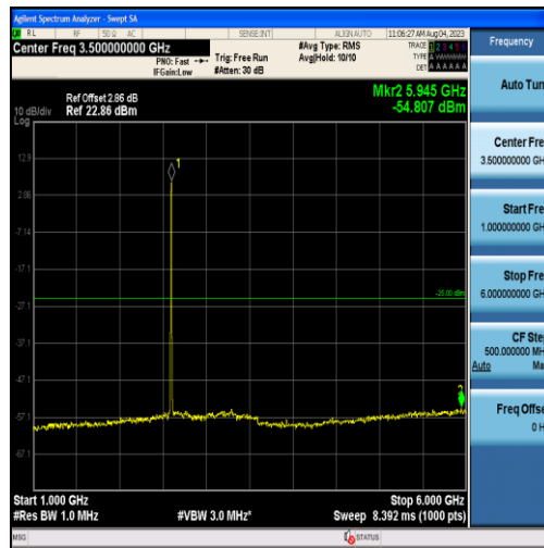
Band38-5MHz-QPSK-38000-25RB#0-Range2:1000~6000MHz
