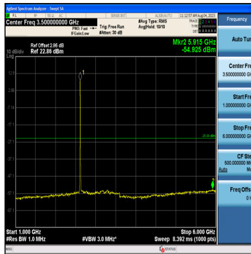
Band38-5MHz-QPSK-38225-25RB#0-Range2:1000~6000MHz
