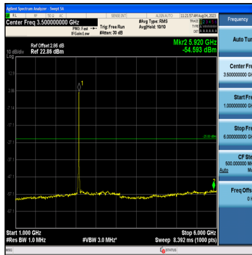
Band38-10MHz-QPSK-37800-50RB#0-Range2:1000~6000MHz
