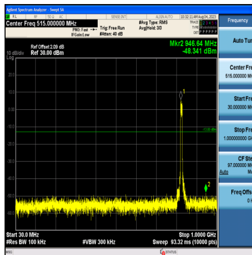
Band26-10MHz-QPSK-26840-50RB#0-Range1:30~1000MHz
