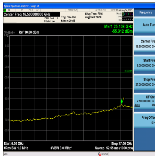
Band38-5MHz-QPSK-38000-25RB#0-Range3:6000~27000MHz
