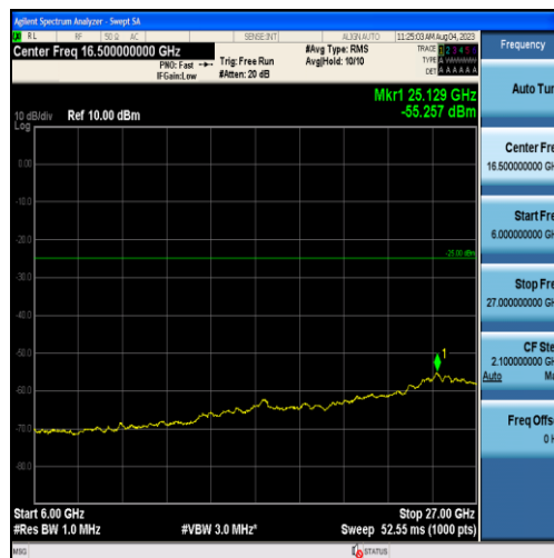
Band38-10MHz-QPSK-37800-50RB#0-Range3:6000~27000MHz
