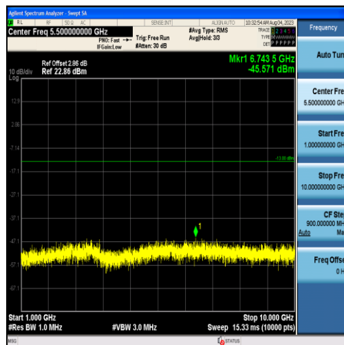
Band26-10MHz-QPSK-26990-50RB#0-Range2:1000~10000MHz
