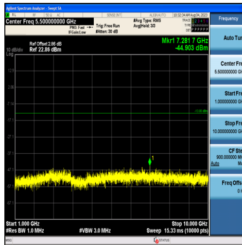
Band26-10MHz-QPSK-26915-50RB#0-Range2:1000~10000MHz
