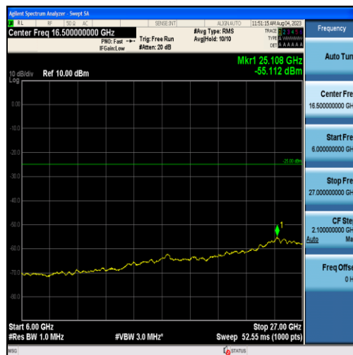
Band38-20MHz-QPSK-37850-100RB#0-Range3:6000~27000MHz
