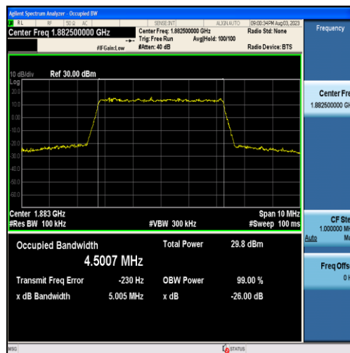
Band25-5MHz-QPSK-26365-25RB#0-4.5007
