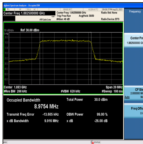
Band25-10MHz-QPSK-26365-50RB#0-8.9754
