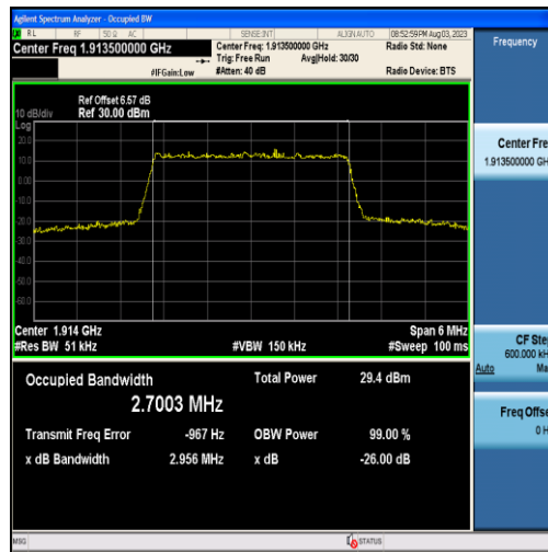
Band25-3MHz-QPSK-26675-15RB#0-2.7003
