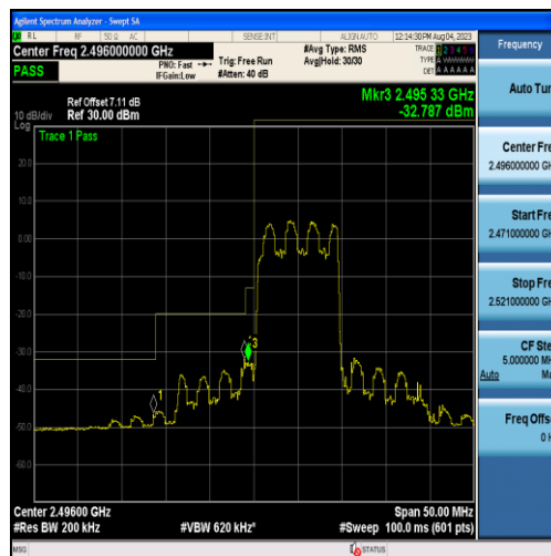
Band41-10MHz-QPSK-39700-50RB#0
