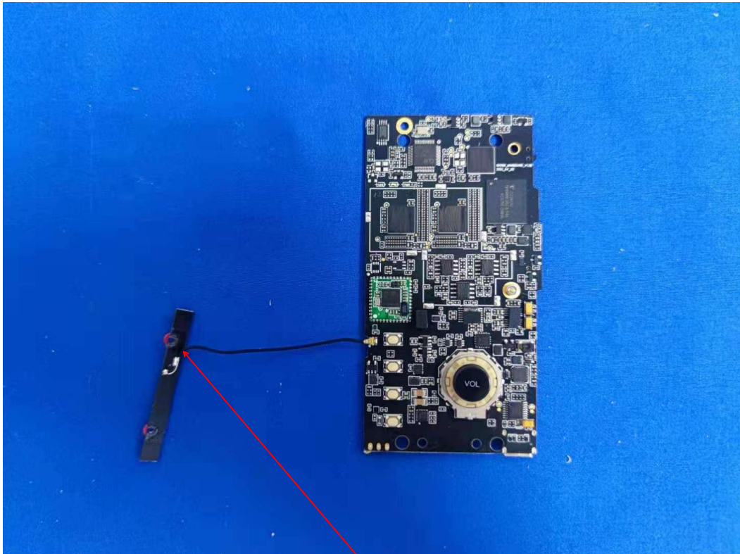
PIFA ANTENNA
