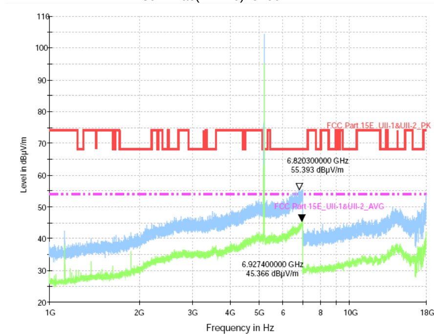
802.11ac(VHT20) 5200MHz
