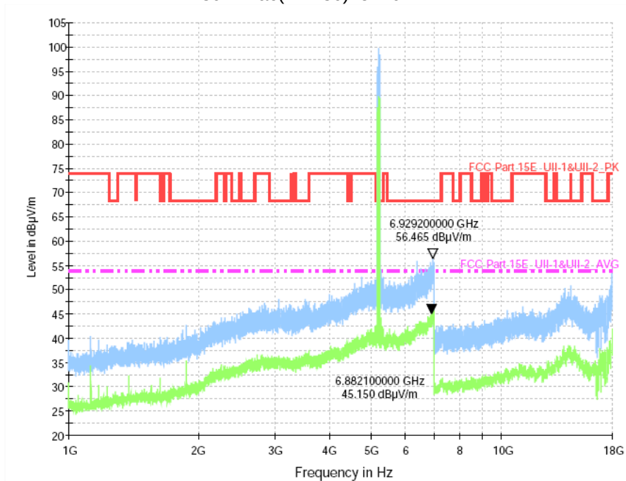
802.11ac(VHT80) 5210MHz
