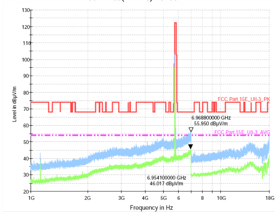
802.11ac(VHT40) 5755MHz
