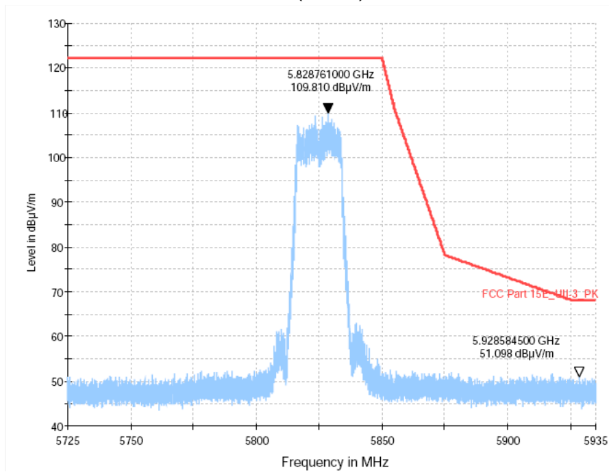
802.11ac(VHT20) HCH
