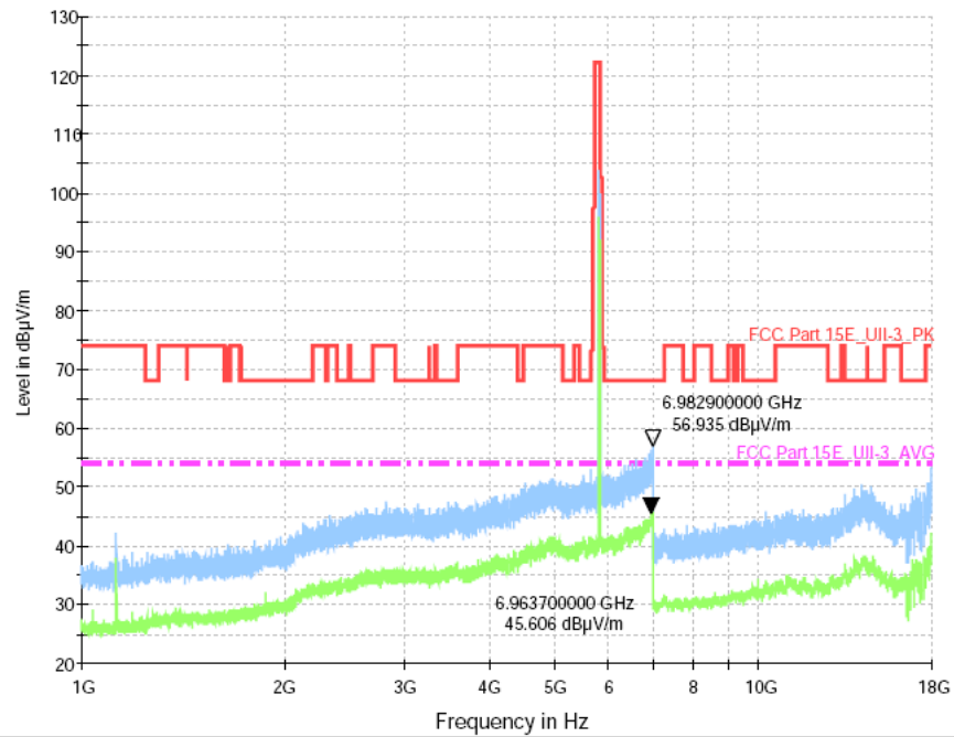
802.11ac(VHT40) 5755MHz
