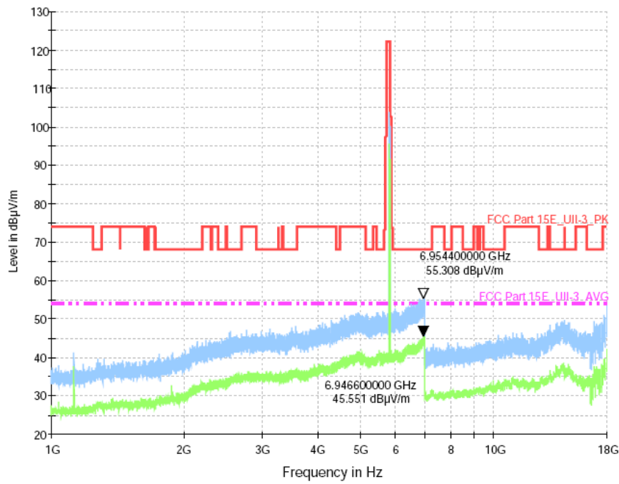
802.11ac(VHT40) 5755MHz
