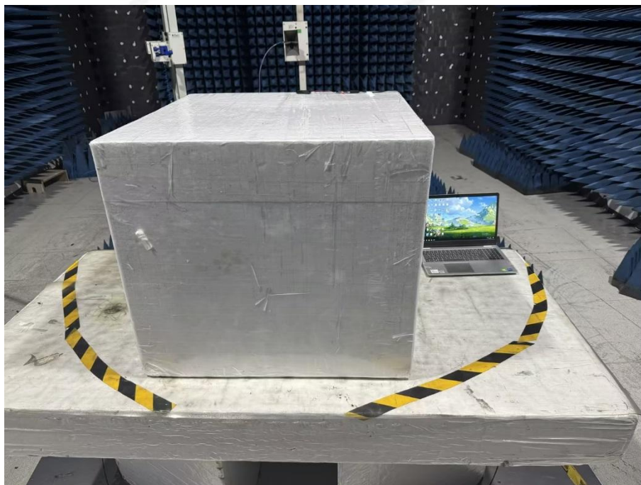
RE (1GHz - 18GHz)
