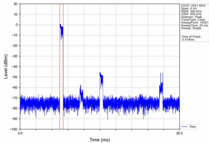
Pi/4DQPSK_2DH1_HOPP_Ant1_NTNV
